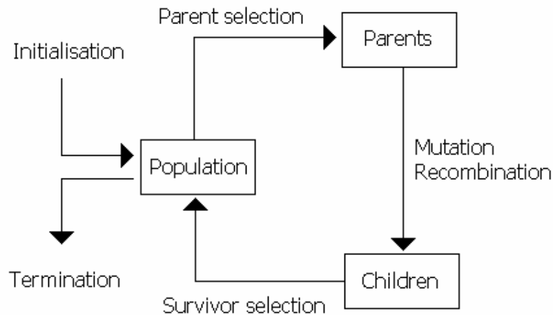
Figuur 46: Schematisch genetisch algoritme
