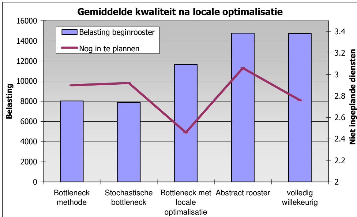
Figuur 42: Gemiddelde kwaliteit na het uitvoeren van lokale optimalisatie
