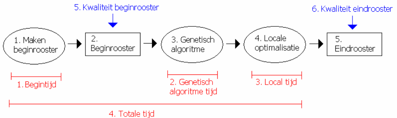
Figuur 43: De onderdelen voor het maken van een rooster
