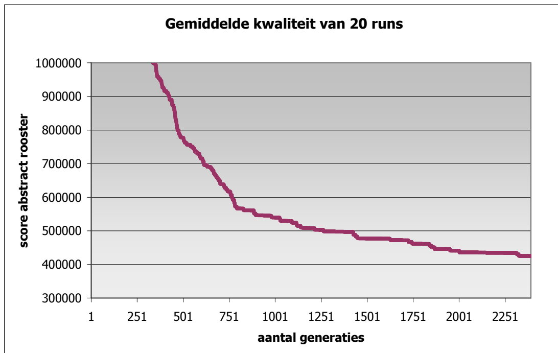
Figuur 29: Kwaliteit per generatie
