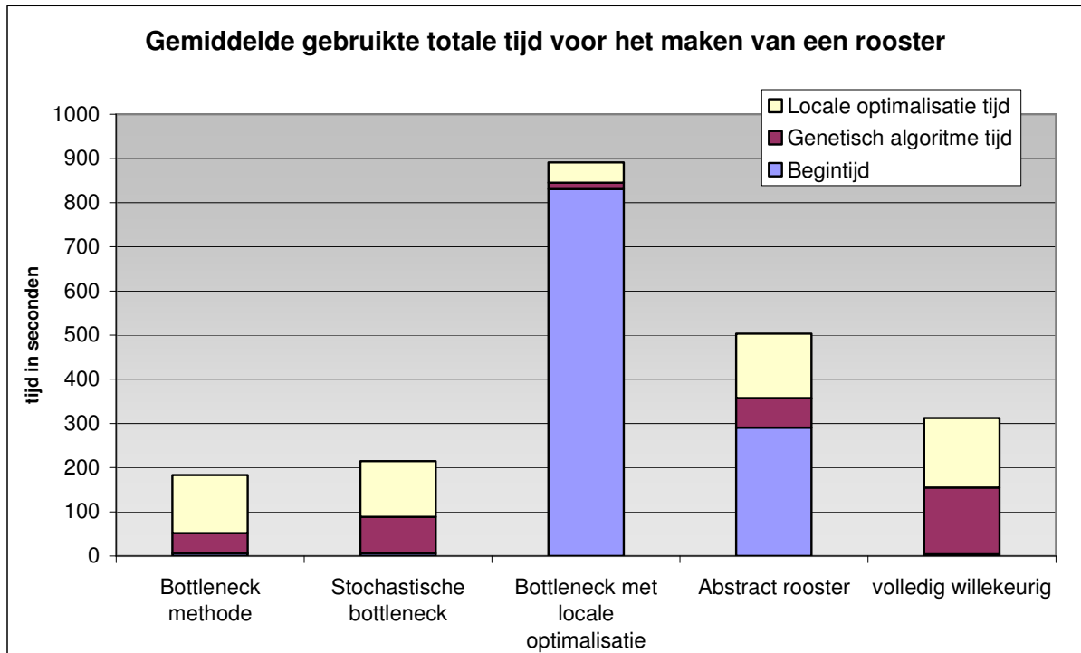
Figuur 38: Gebruikte tijd voor het maken van een rooster
