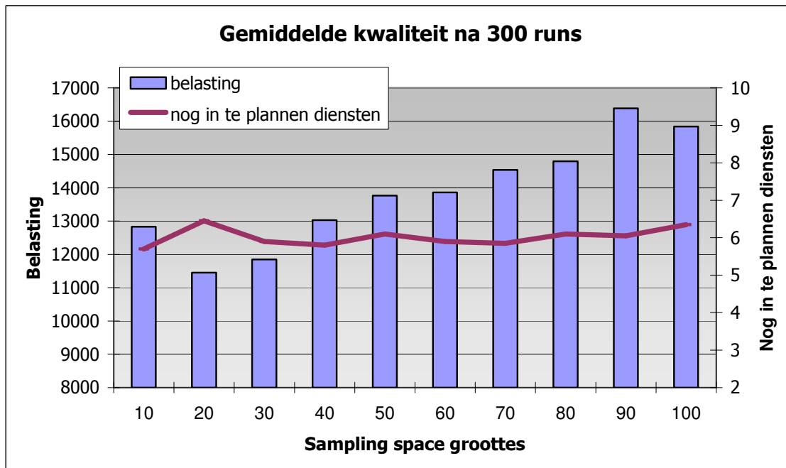
Figuur 19: Test van kwaliteit bij verschillende sampling space groottes
