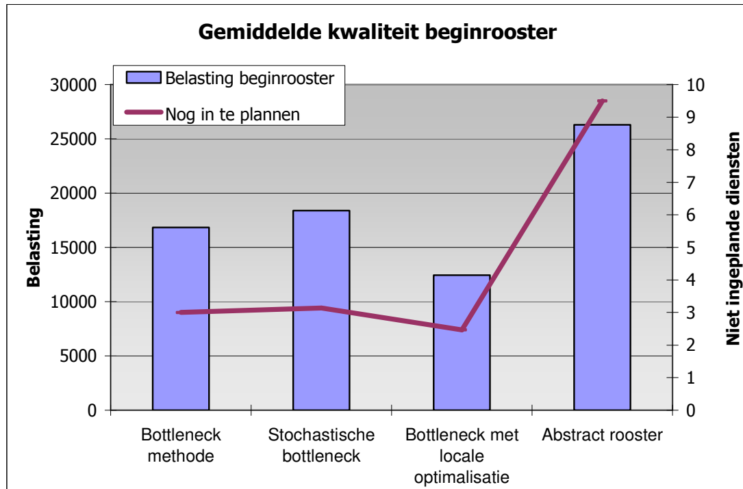
Figuur 40: Gemiddelde kwaliteit van het beste beginrooster van de vijf die zijn gemaakt 3
