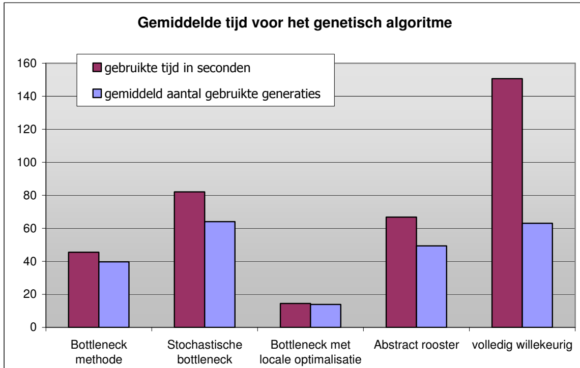
Figuur 36: Gemiddelde tijd nodig voor het uitvoeren van het genetisch algoritme over 100 runs
