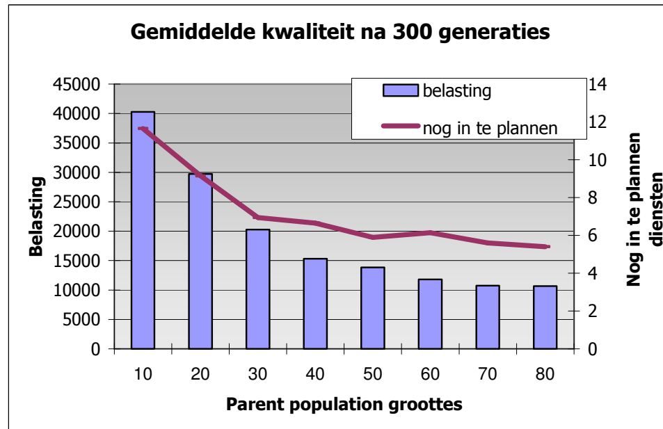
Figuur 22: Kwaliteit na 300 generaties bij verschillende parent population groottes
