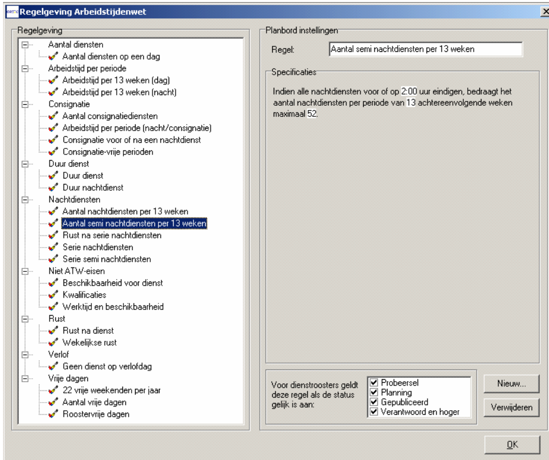
Figuur 45: Regelgeving HARMONY
