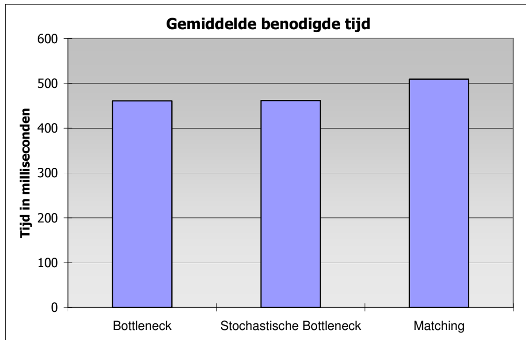
Figuur 33: Benodigde tijd voor het uitvoeren van 300 generaties
