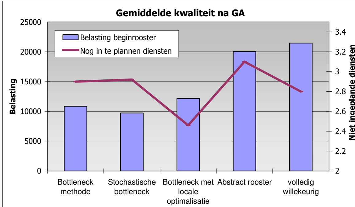
Figuur 41: Gemiddelde kwaliteit na het uitvoeren van het genetisch algoritme
