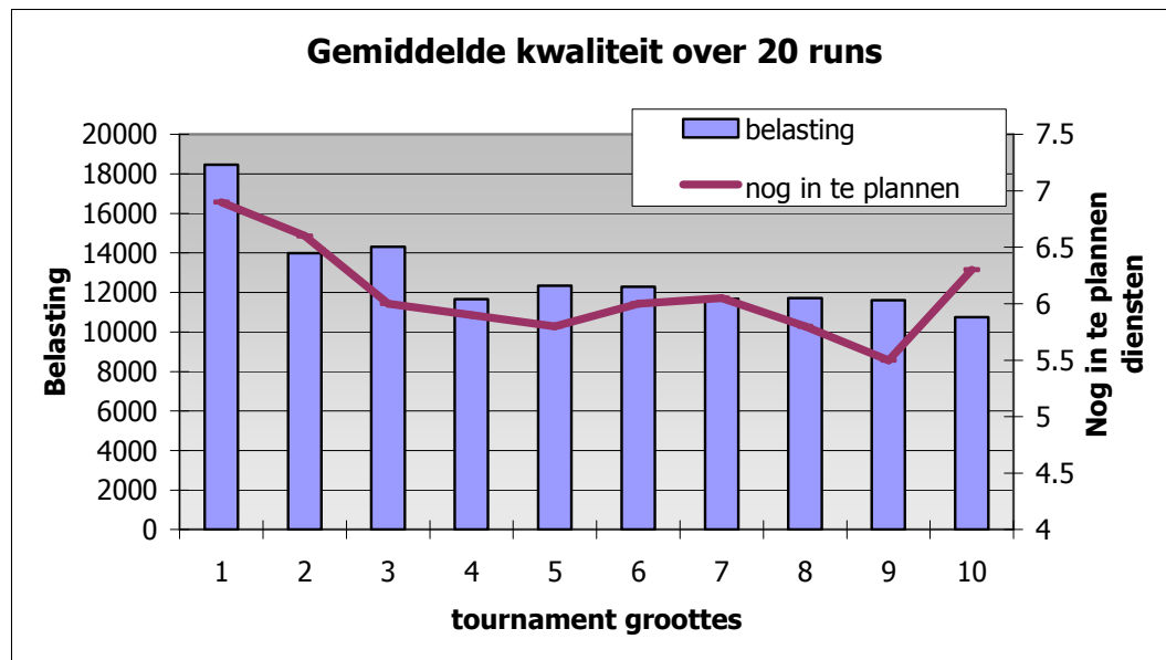
Figuur 26: Gemiddelde kwaliteit bij verschillende tournament groottes
