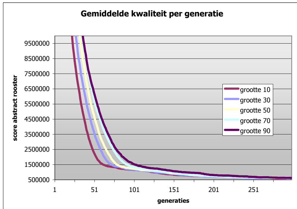
Figuur 20: Gemiddelde kwaliteit per generatie voor 20 runs
