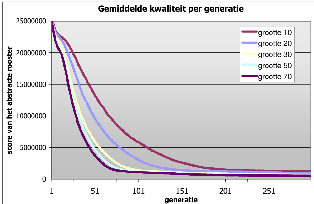
Figuur 23: Gemiddelde kwaliteit per generatie voor verschillende parent population groottes
