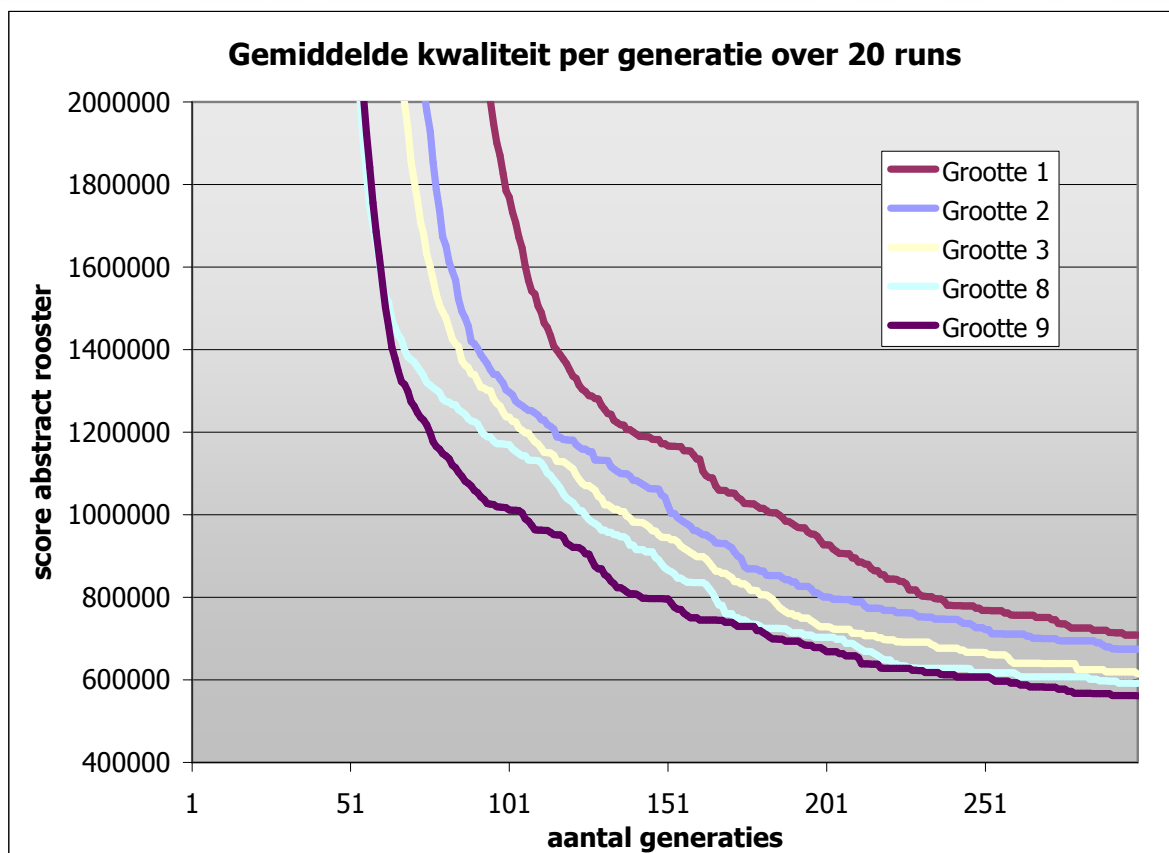
Figuur 27: Kwaliteit per generatie bij verschillende tournament groottes
