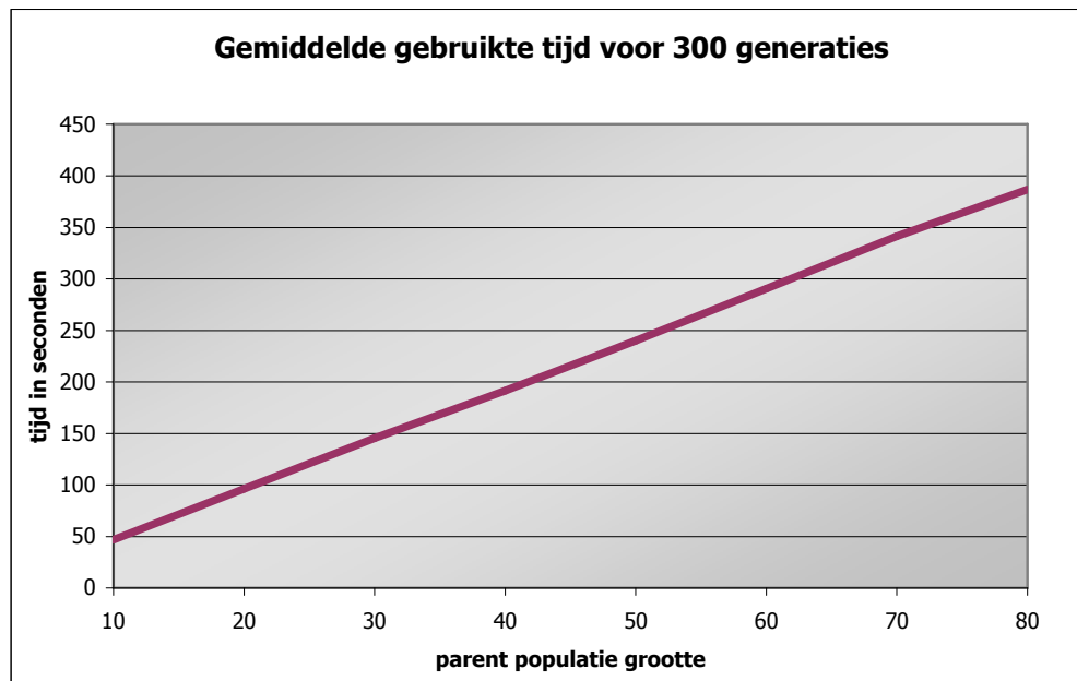
Figuur 25: Gemiddelde benodigde tijd voor het maken uitvoeren van 300 generaties
