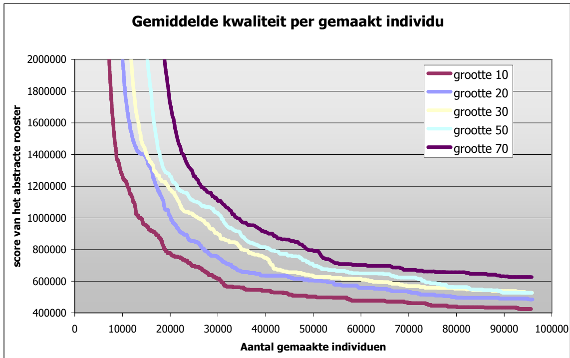
Figuur 24: kwaliteit per gemaakt individu
