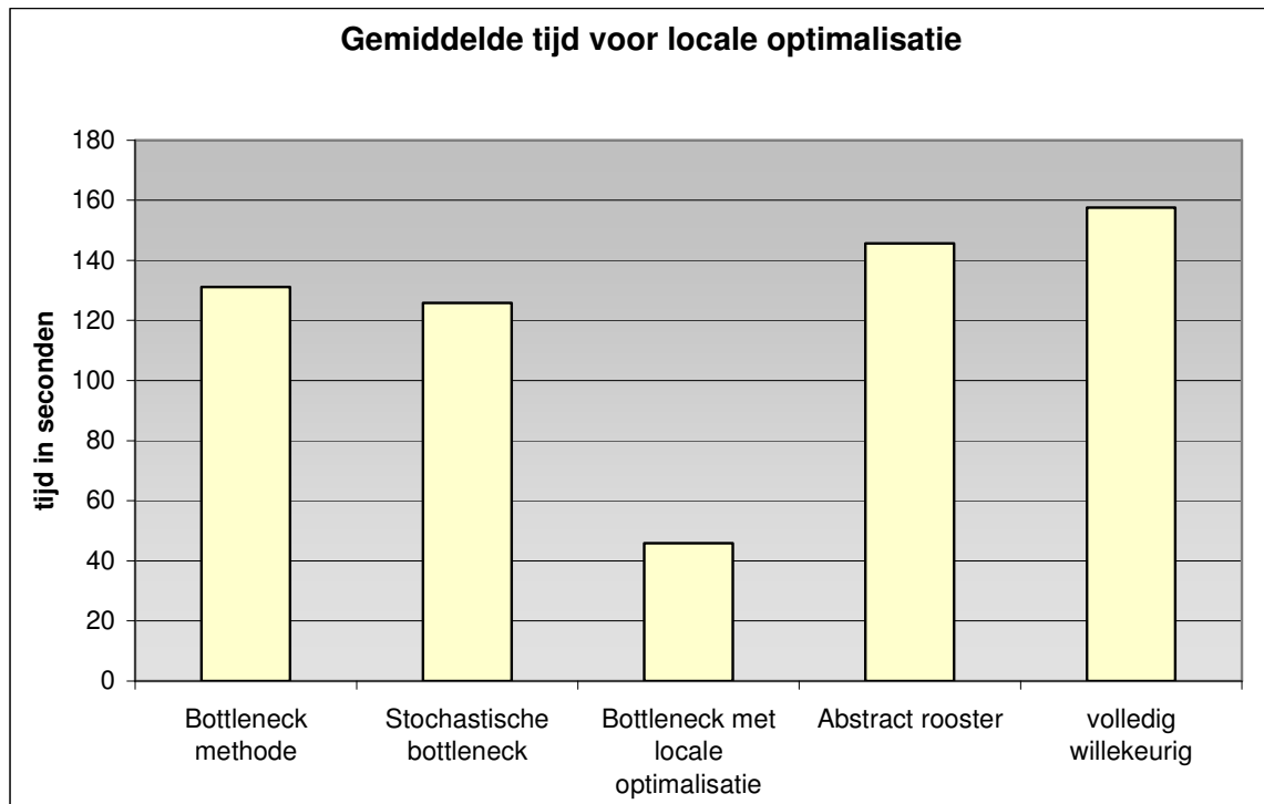
Figuur 37: Gemiddelde tijd gebruikt voor lokale optimalisatie
