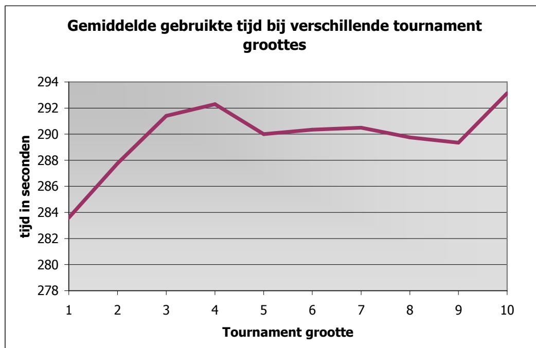
Figuur 28: Gebruikte tijd voor het uitvoeren van 300 generaties bij verschillende tournament groottes
