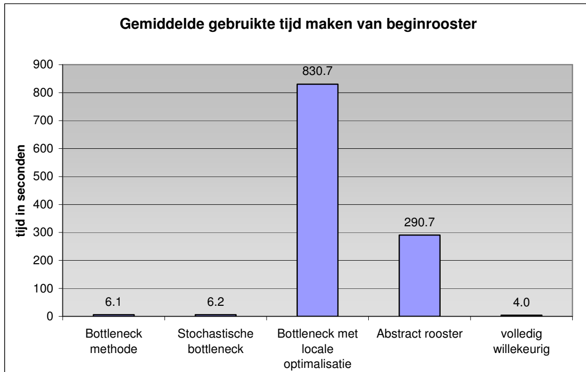
Figuur 35: gemiddelde gebruikte tijd voor het maken van een beginrooster per methode
